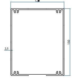
Profile No kg/m YNG-6569 3,994
