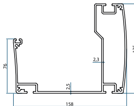
Profile No kg/m YNG-5935 3,918
