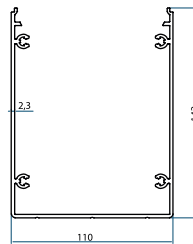
Profile No kg/m YNG-2301 3,003
