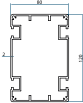
Profile No kg/m YNG-5936 3,032
