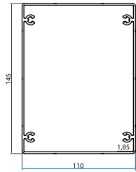
Profile No kg/m YNG-2111 3,044
