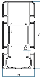
Profile No kg/m YNG-6413 4,655
