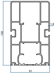
Profile No kg/m YNG-2052 5,217
