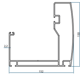
Profile No kg/m YNG-2078 4,398
