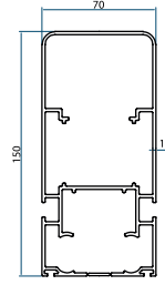
Profile No kg/m YNG-2156 3,217
