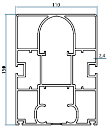
Profile No kg/m YNG-2001 7,168
