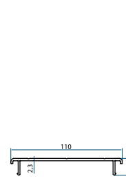
Profile No kg/m YNG-2302 0,846
