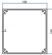
Profile No kg/m YNG-6565 2,463
